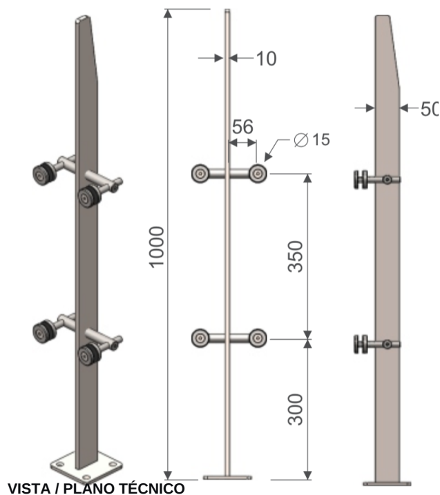
VISTA / PLANO TÉCNICO
