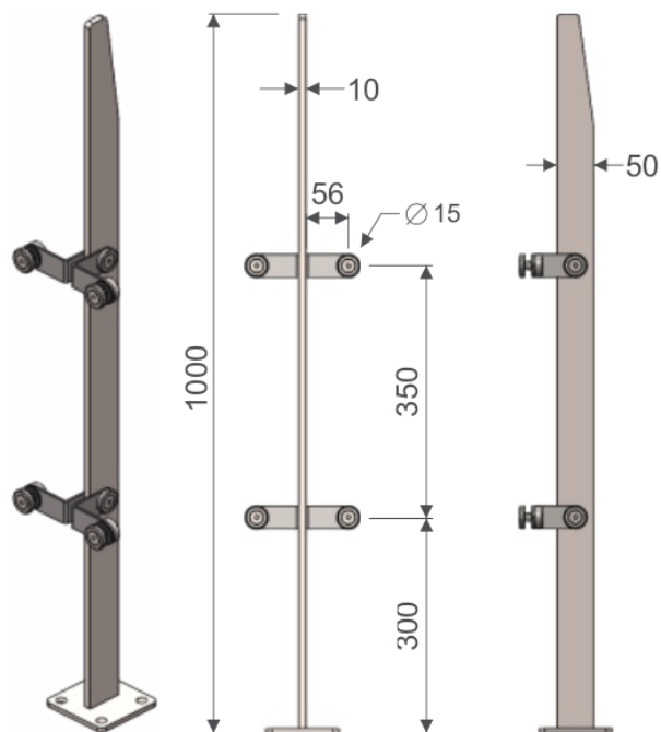
VISTA / PLANO TÉCNICO
