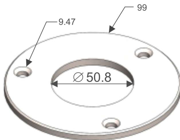
VISTA / PLANO TÉCNICO
