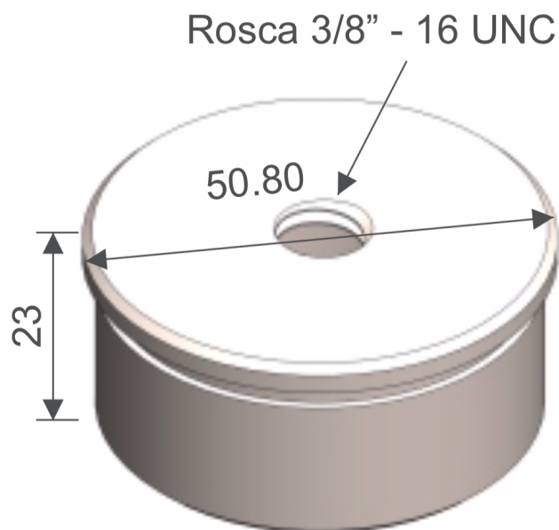
VISTA / PLANO TÉCNICO
