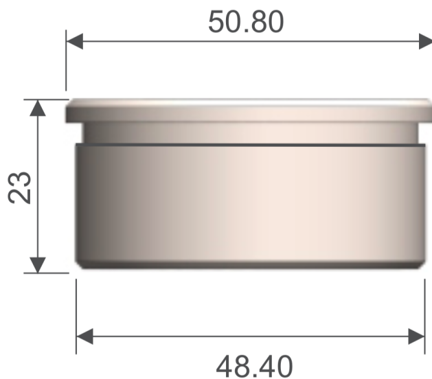
VISTA / PLANO TÉCNICO
