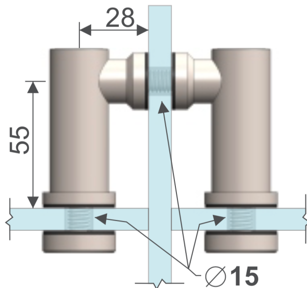
VISTA / PLANO TÉCNICO
